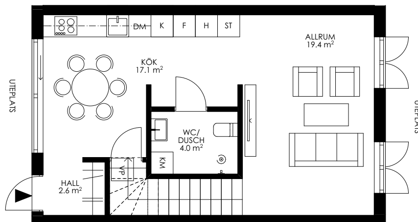
ENTRÉPLAN
