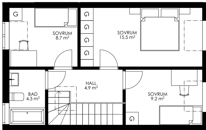
ÖVRE PLAN
