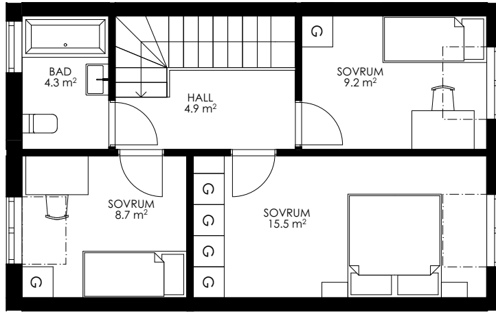
ÖVRE PLAN
