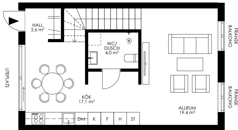
ENTRÉPLAN
