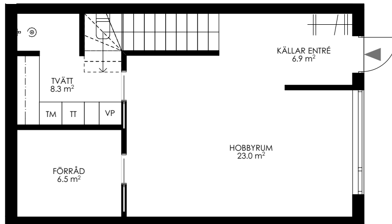
KÄLLARPLAN
