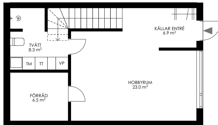
KÄLLARPLAN
